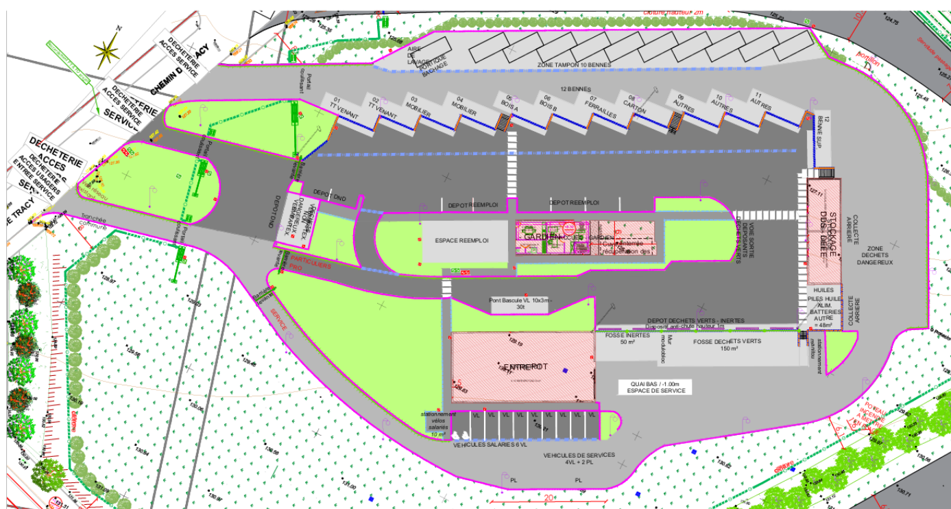
Schéma de la nouvelle déchèterie
